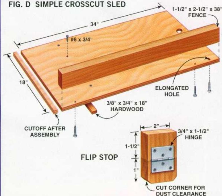
FIG. D SIMPLE CROSSCUT SLED
