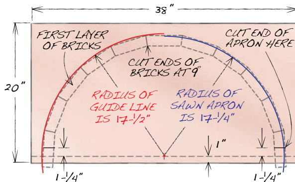
Fig. B Apron Staging Board
