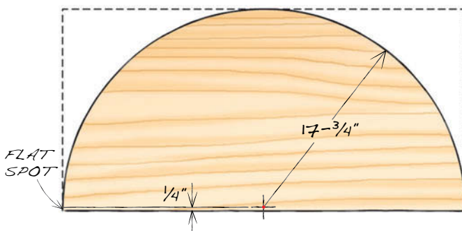
Fig. M Top Layout
