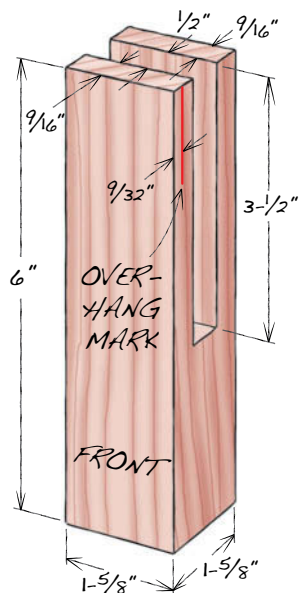
Fig. E Leg Gauge
