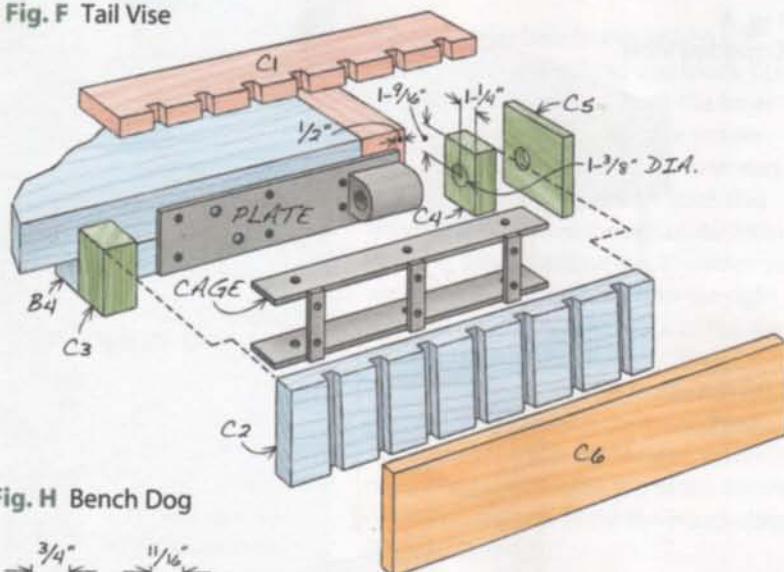
Fig. F Tail Vise
