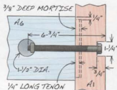
Fig. E End Cap Bolts
